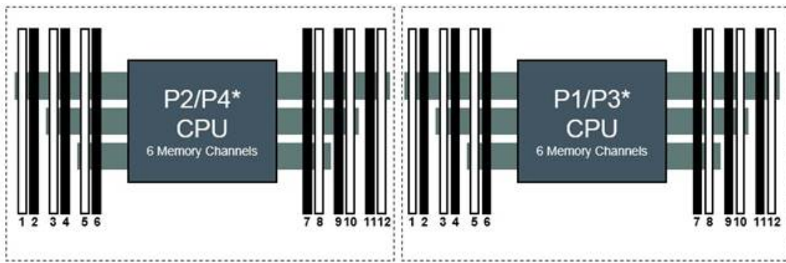
HPE Gen10 DL360 / DL380 / DL560
