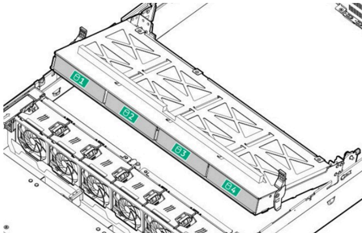
4 LFF Mid Tray
