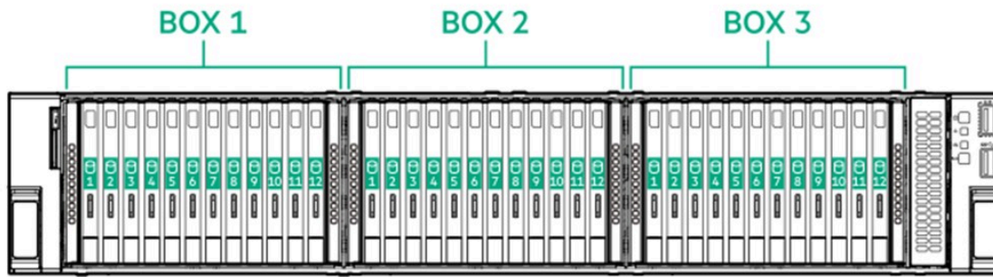
36 EDSFF E3.S 1T Drives
