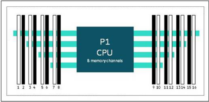
HPE ProLiant DL320 Gen10 Plus
